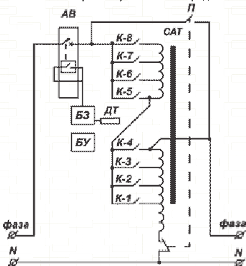
Рис.1 Релейный тип стабилизации
