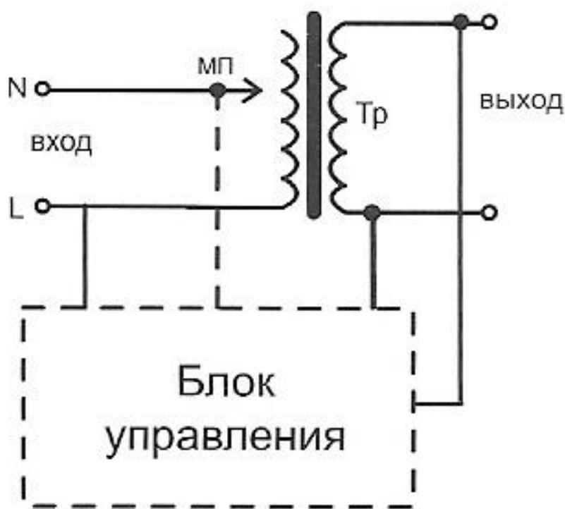
Рис.2 Электромеханический тип стабилизации
