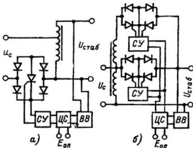
Рис. 3 Схема с двусторонним ключом на одном тиристоре
