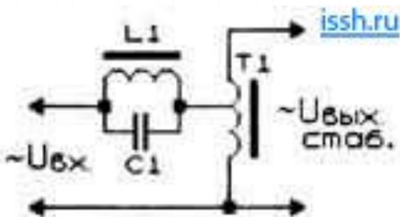
Рис. 5. Схема феррорезонансного стабилизатора с дросселем насыщения
